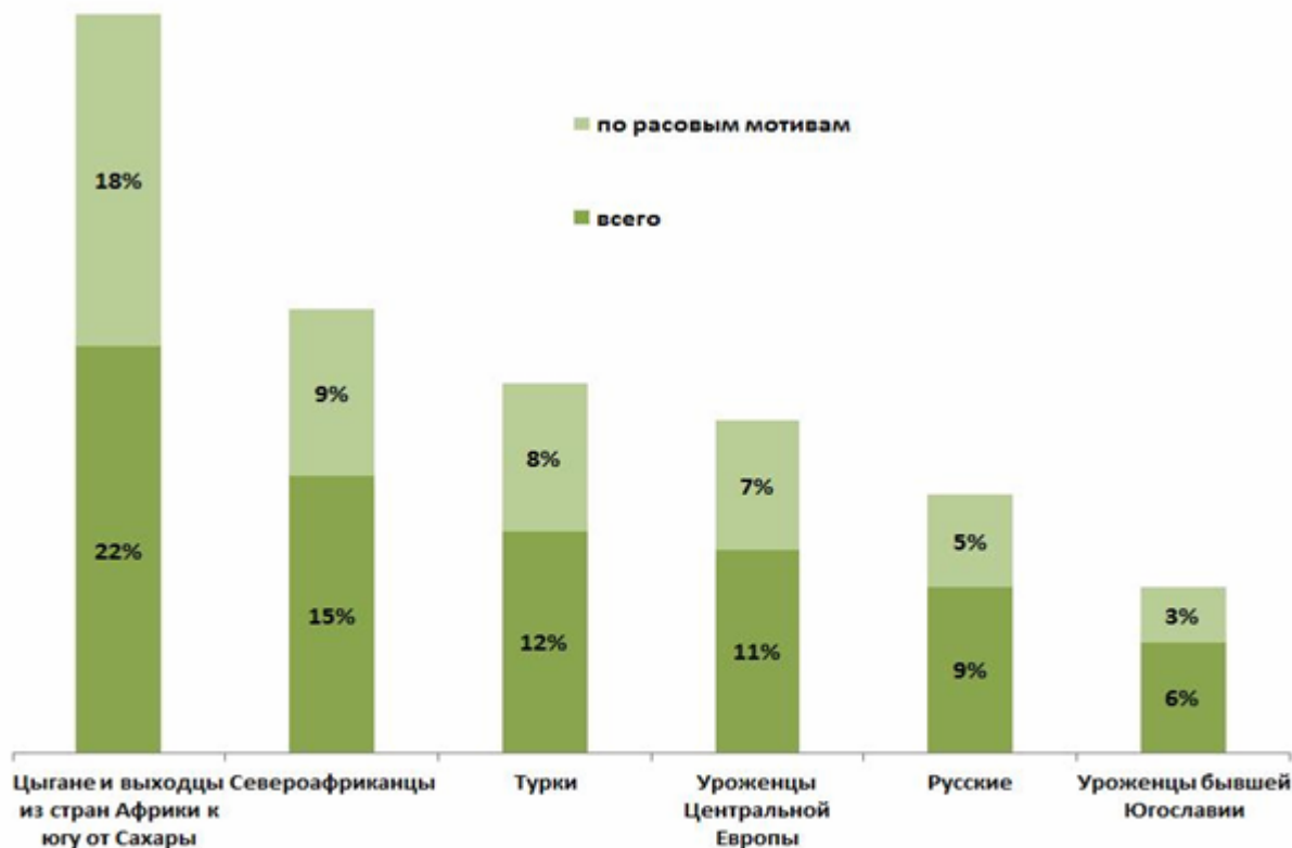
Рисунок 2 – Национальный состав жертв экстремизма в странах ЕС в период с 2001 – 2007 гг., %
